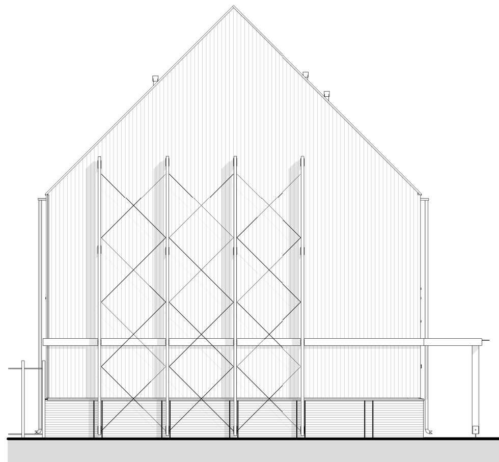
kopgevel (zuid)
