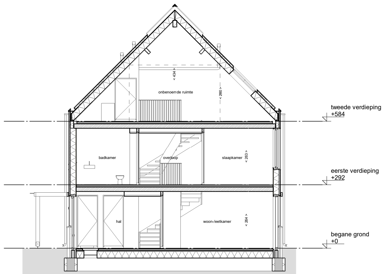
doorsnede
