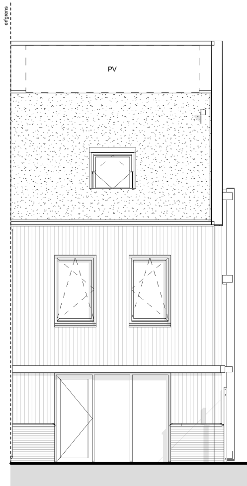
achtergevel (west)
